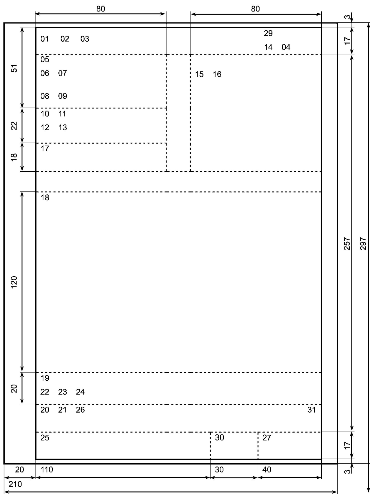
Рисунок Б.1 - Расположение реквизитов и границы зон
